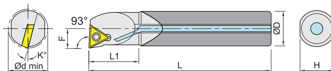
Coolant carbide shank (Right-hand shown) 中心出水鎢鋼柄 右向示意圖
