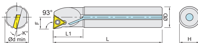
Coolant steel shank (Right-hand shown) 中心出水鋼柄 右向示意圖
