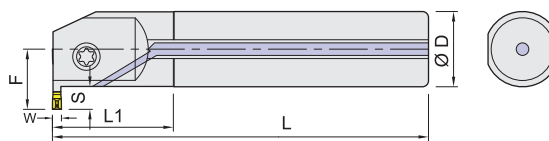
Coolant steel shank (Right-hand shown) 中心出水鋼柄 右向示意圖
